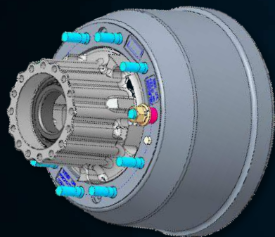
CONJ. CUBO E TAMBOR TRASEIRO
