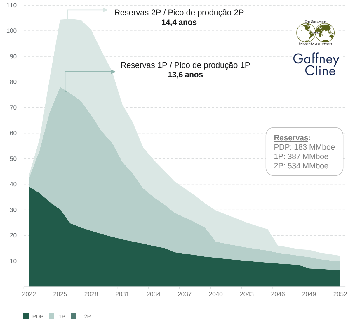
Produção futura estimada de O&G de ativos 3R 2 (kboe/dia) | Estimativas dos relatórios de certificação elaborados pela Degolyer and MacNaughton e GaffneyCline
